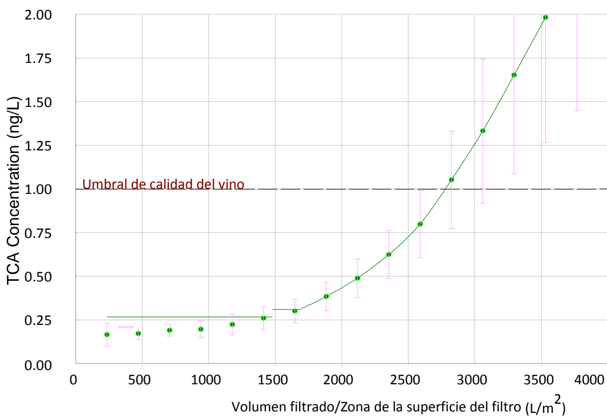
Eficacia de las placas de filtración en profundidad con zeolita Y-faujasita Curva de ruptura del TCA 3
